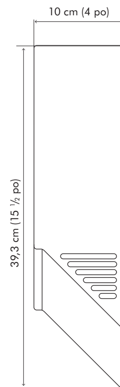
ÉLÉVATION LATÉRALE
