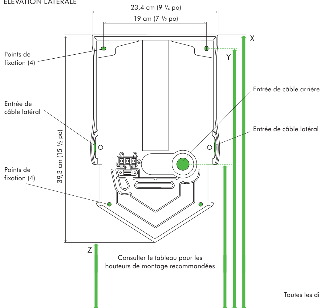
ÉLÉVATION LATÉRALE
